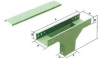
上边垂直等径三通XQJ-C-03D
