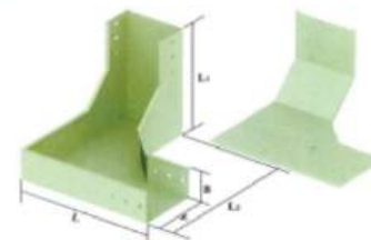
垂直下弯右弯通XQJ-C-DB
