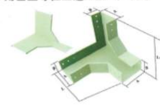
下角垂直等径三通XQJ-C-03G
