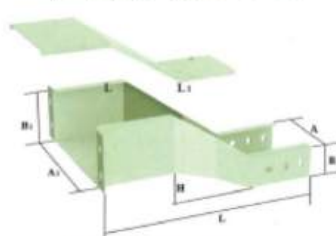
爬低喇叭口XQJ-C-SA
