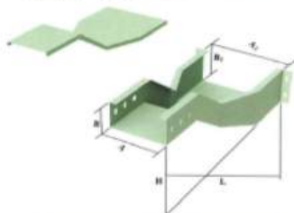
爬高喇叭口XQJ-C-SB
