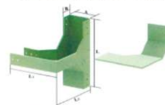
下垂直弯三通XQJ-C-AC
