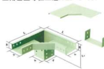
上角垂直等径三通XQJ-C-03F
