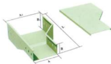
上右平异径接头XQJ-C-05B
