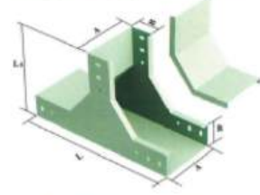
下垂直等径三通XQJ-C-03C
