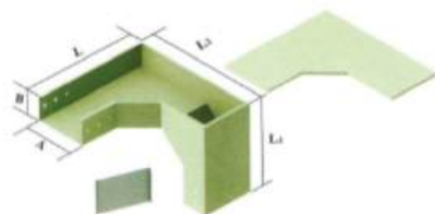
垂直弯右弯通XQJ-C-FB
